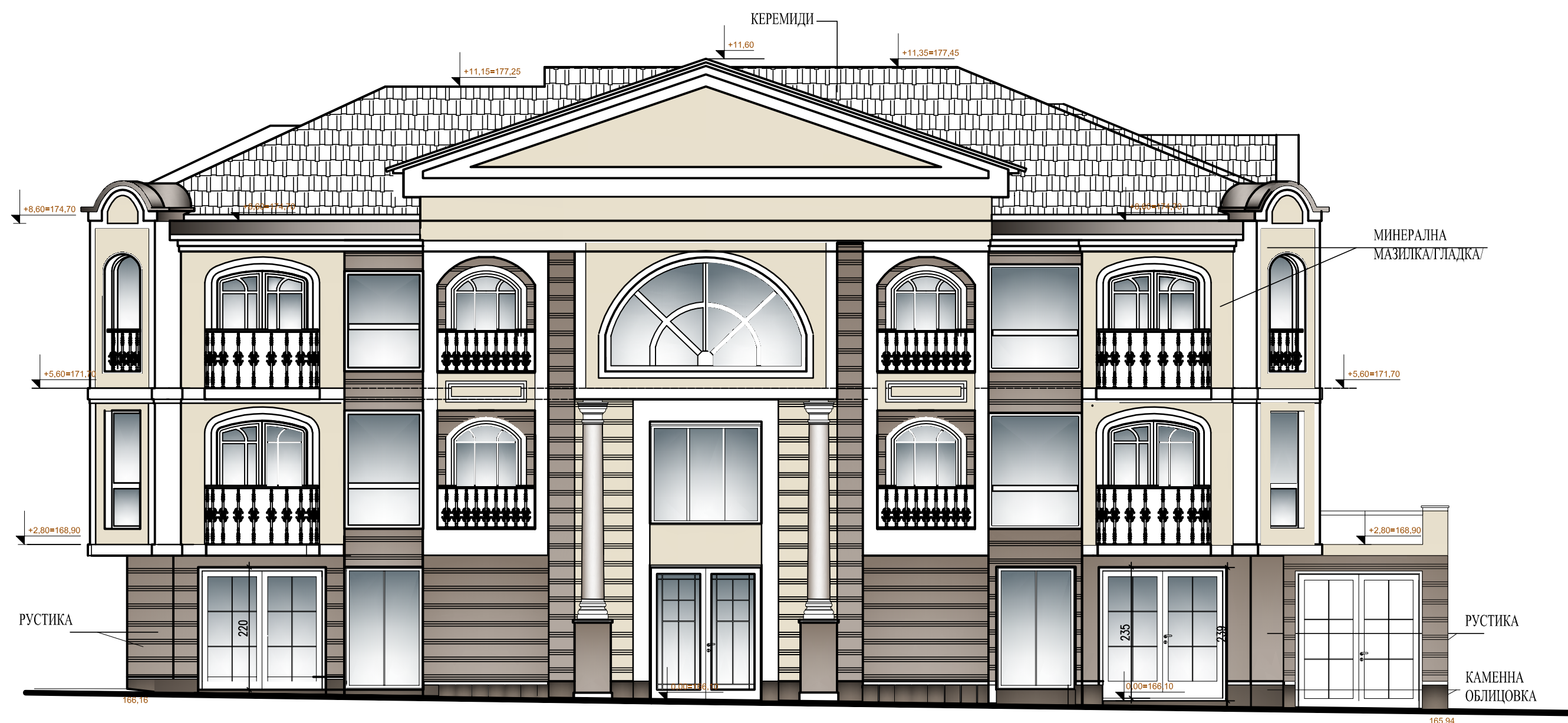
ВАРИАНТ 2 ФАСАДА ЮГОИЗТОК М 1 : 50
